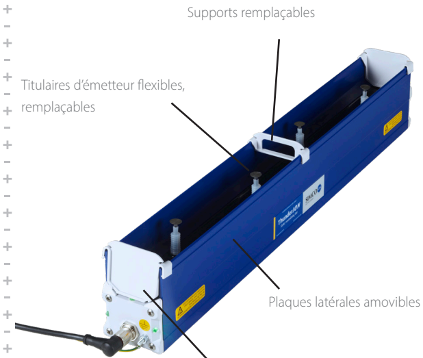
Flasques remplaçables
