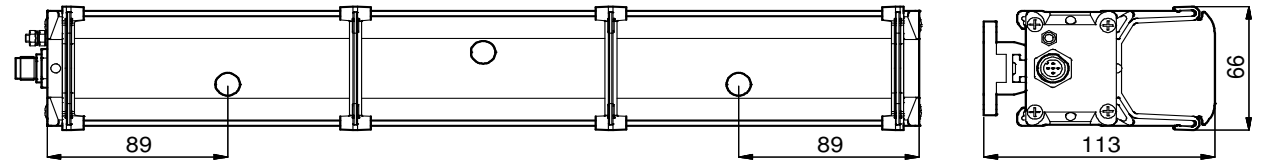
Technische tekening ThunderION IQ 2.0
